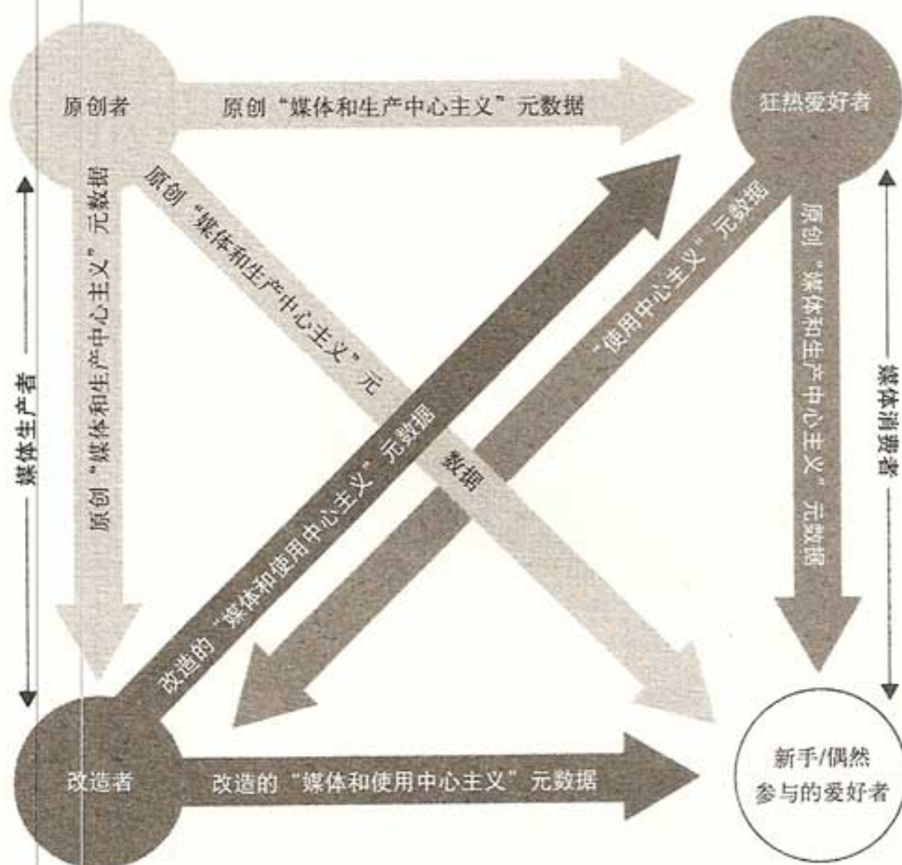
图4-1 参与机制
