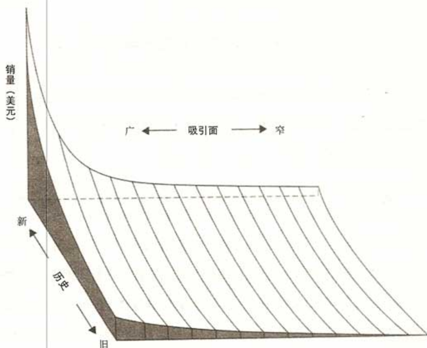
图7-6 时间长尾
