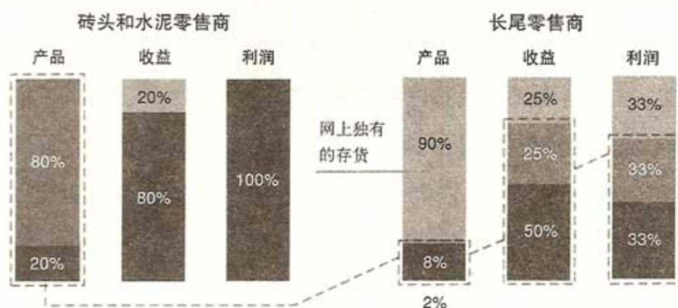
图7-3 80/20法则的演化
