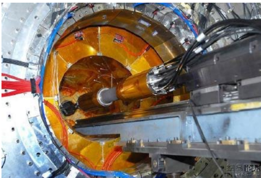
新北谱仪超导螺线管磁体绕线正式开始绕线
