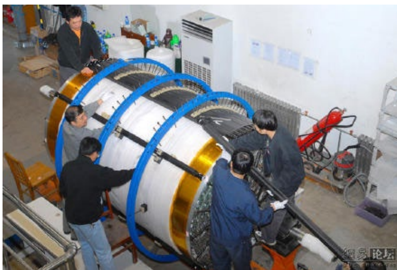
桶部飞行时间探测器由两层 176 个单元组成，每个单元包括塑料闪烁体、光电倍增管和套筒三部分
