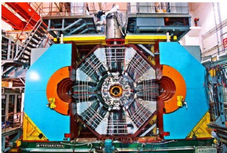
规模巨大的 BESIII 探测器（长 11 米，宽 6 米，高 6.5 米，机械结构总重量达 650 吨）
